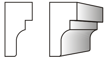
120h x 60w
